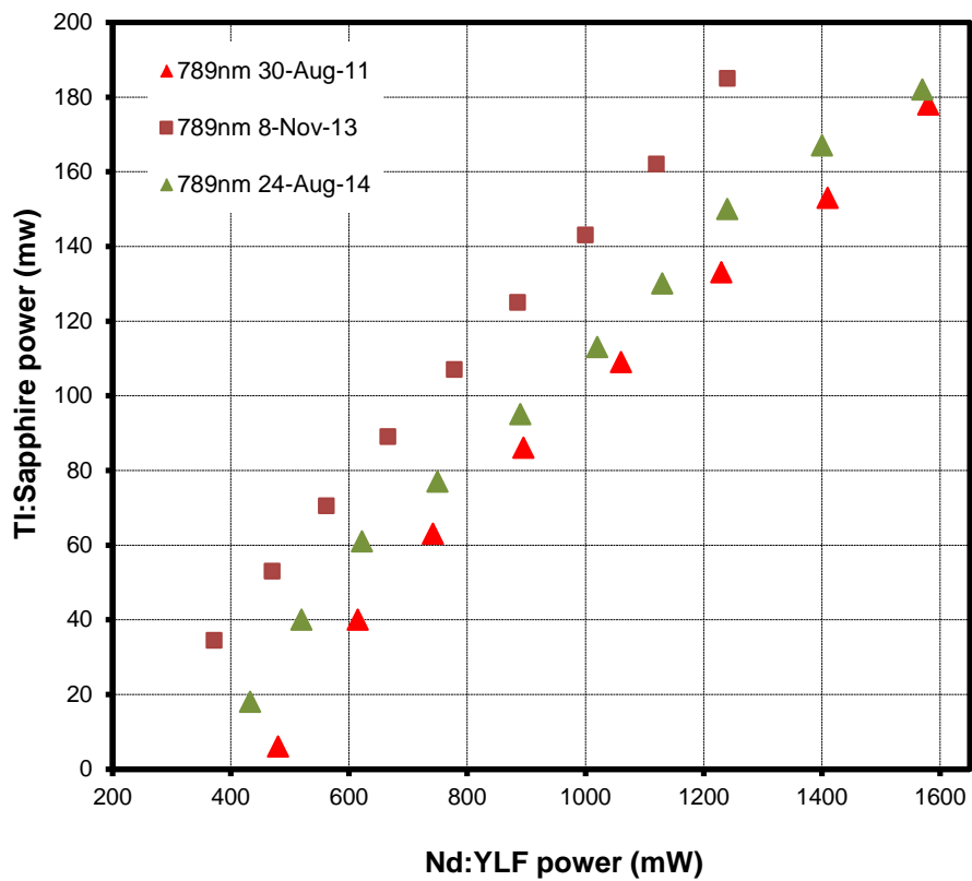
Nd:YLF LASER PUMPED TI:S LASERS 3
