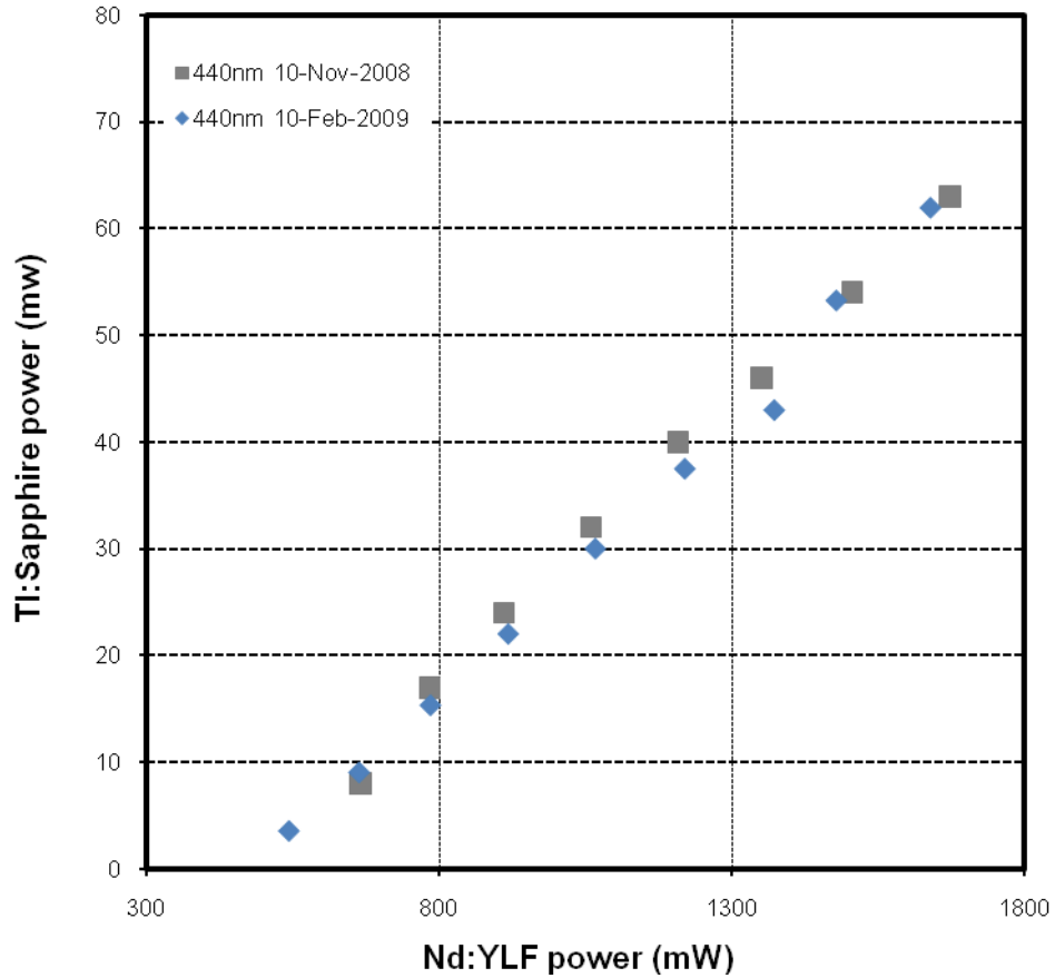
Nd:YLF LASER PUMPED TI:S LASERS 1
