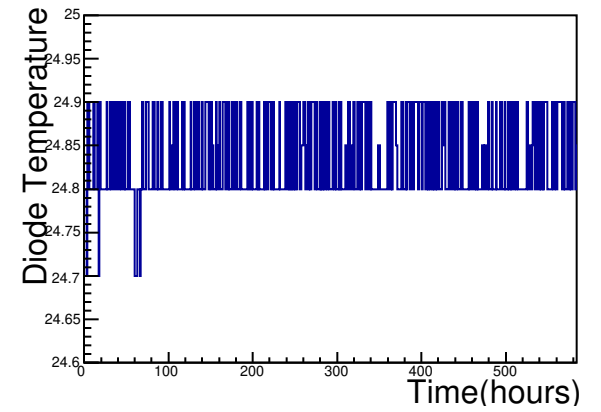
DP2-447 Laser 2
