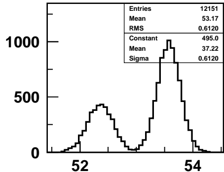
Energy (mJ)
