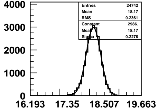
FWHM (ns)
