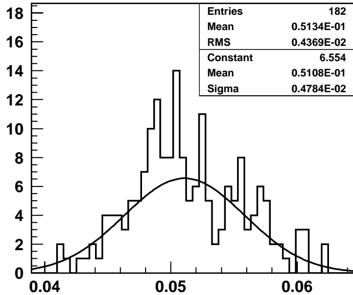
Energy (mJ)
