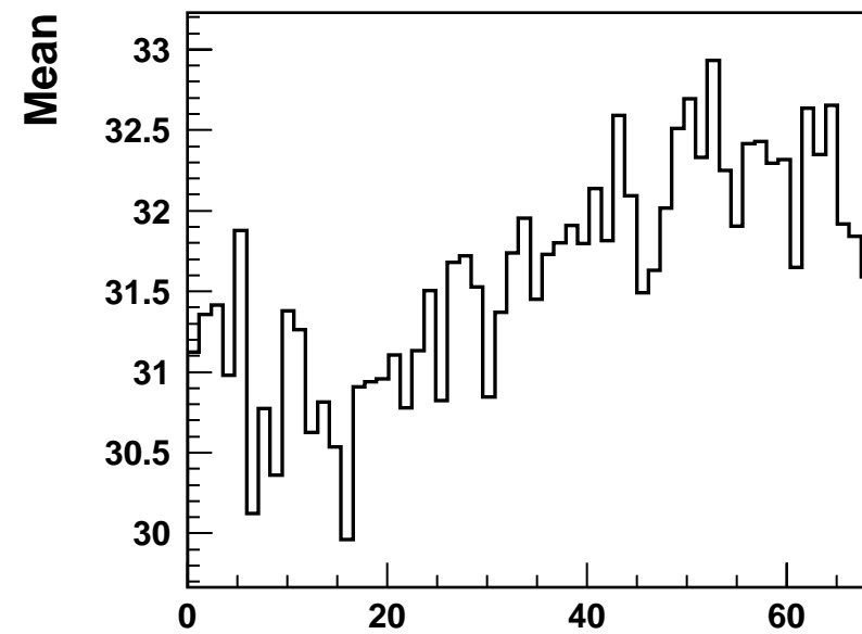
Ti:S Laser
