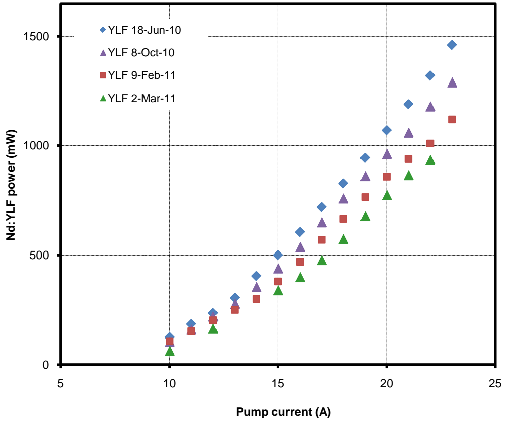
Nd:YLF LASERS 3
