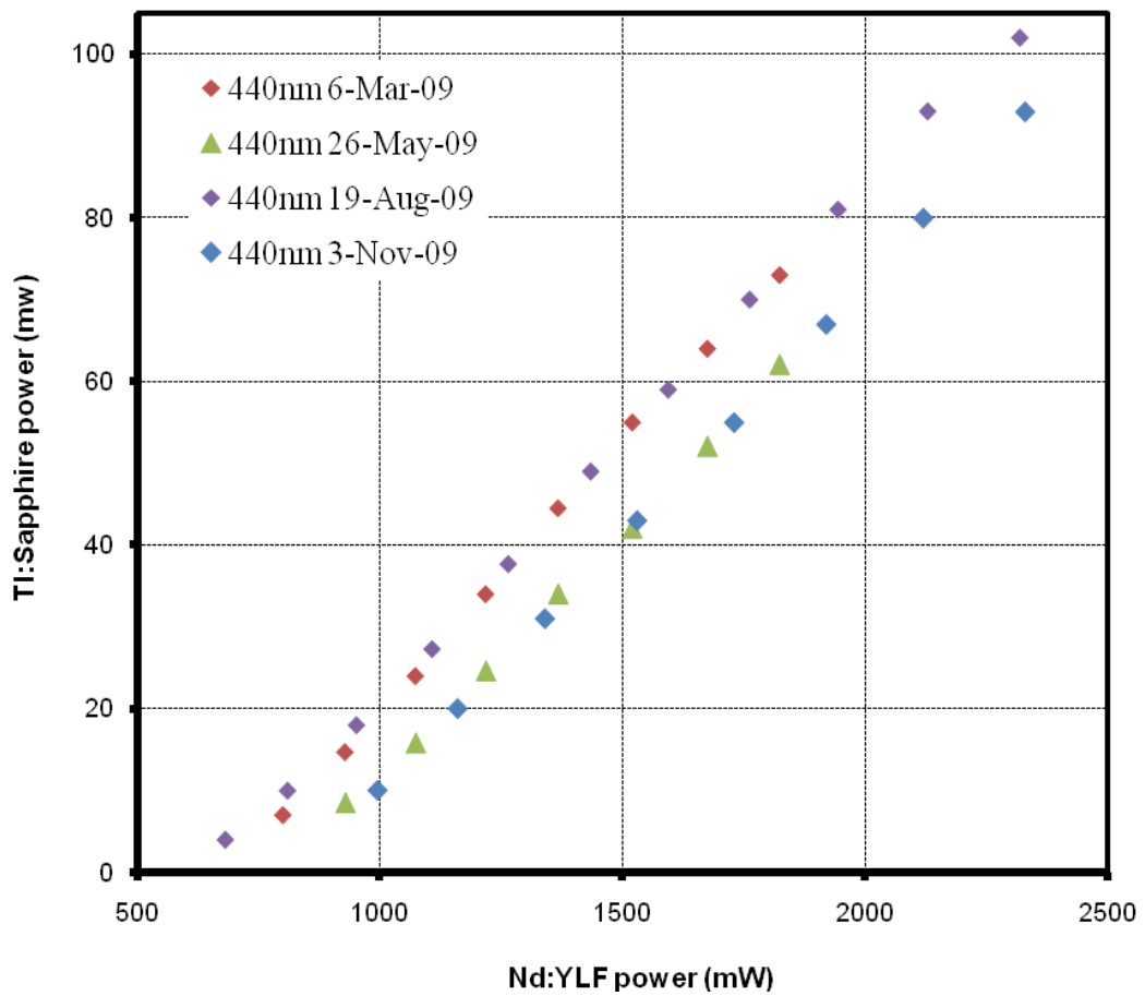
Nd:YLF LASER PUMPED TI:S LASERS 2
