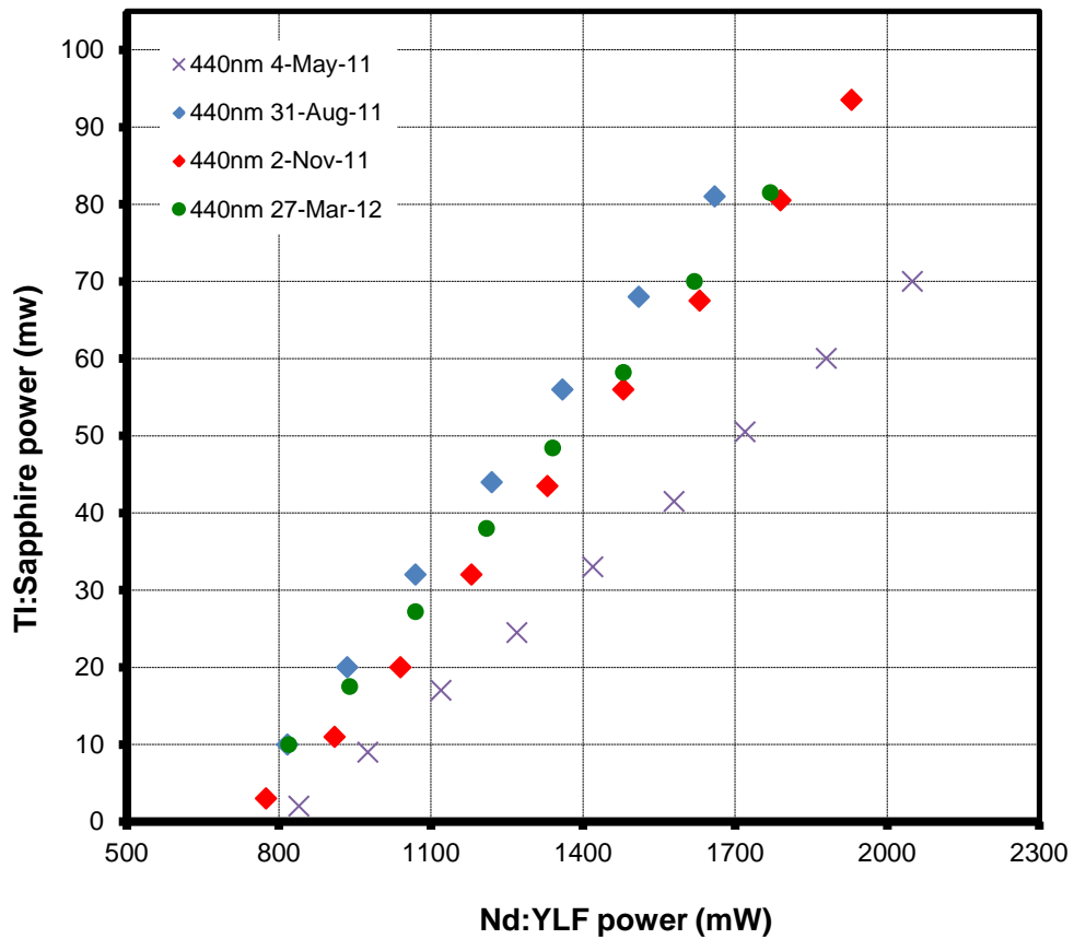
Nd:YLF LASER PUMPED TI:S LASERS 2
