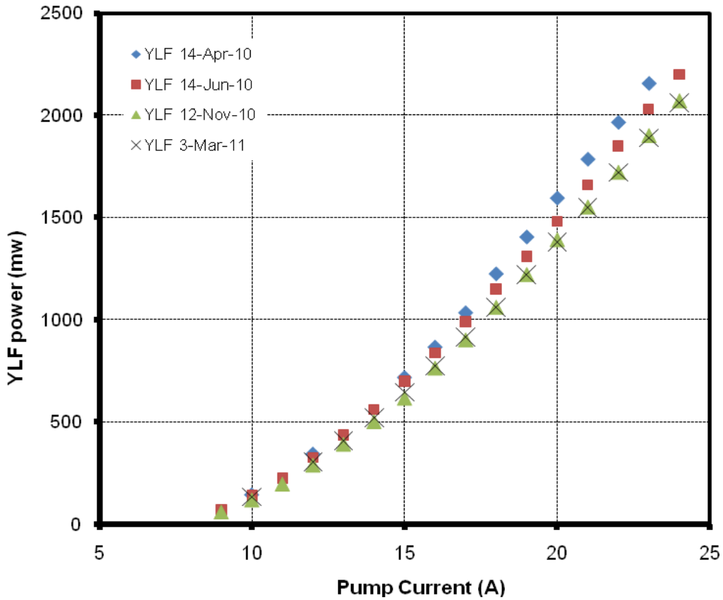
Nd:YLF LASERS 2
