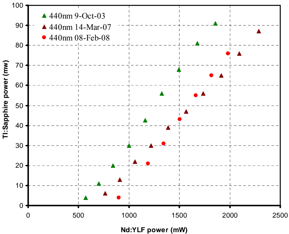
Nd:YLF LASER PUMPED TI:S LASERS 2
