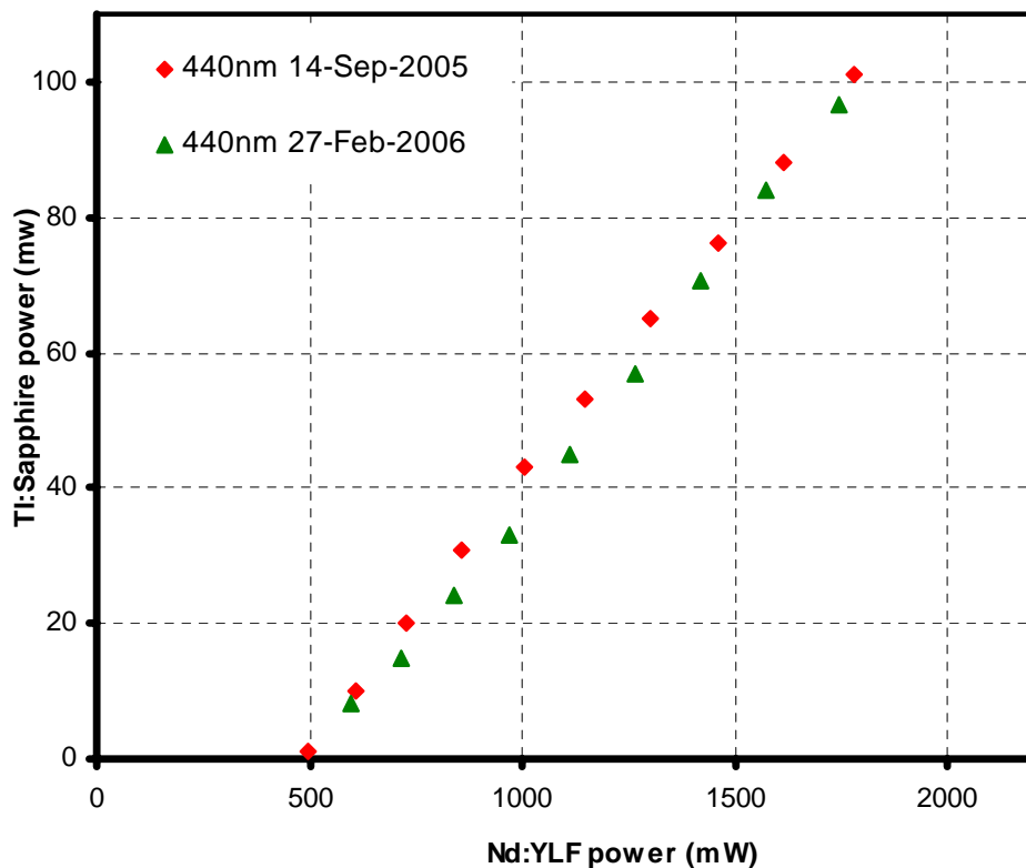
Nd:YLF LASER PUMPED TI:S LASERS 1
