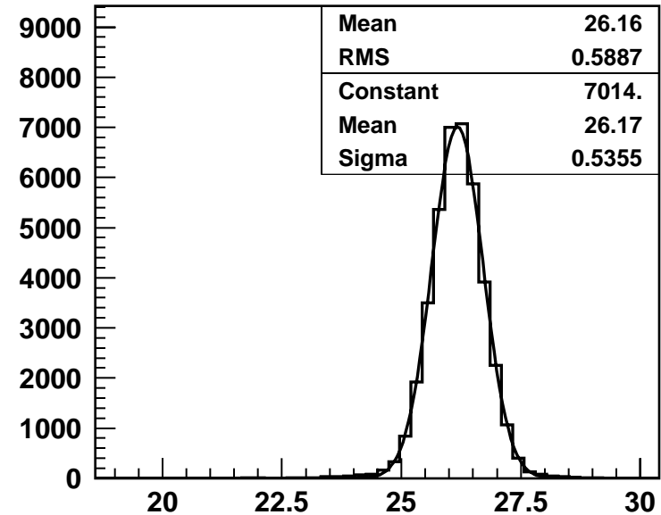
FWHM (ns)
