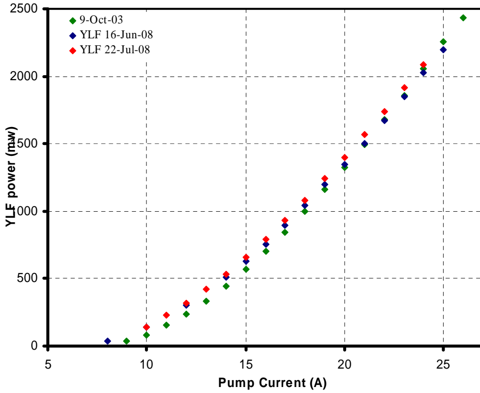
Nd:YLF LASERS 2
