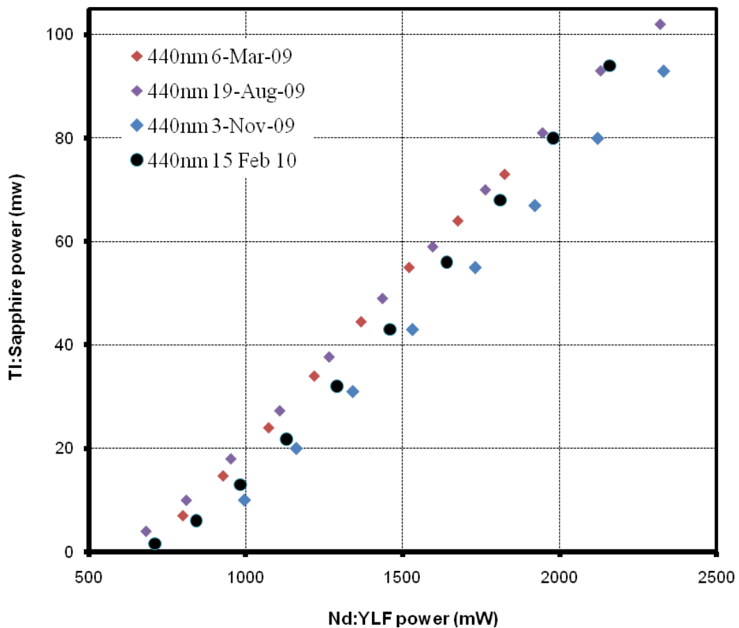
Nd:YLF LASER PUMPED TI:S LASERS 2
