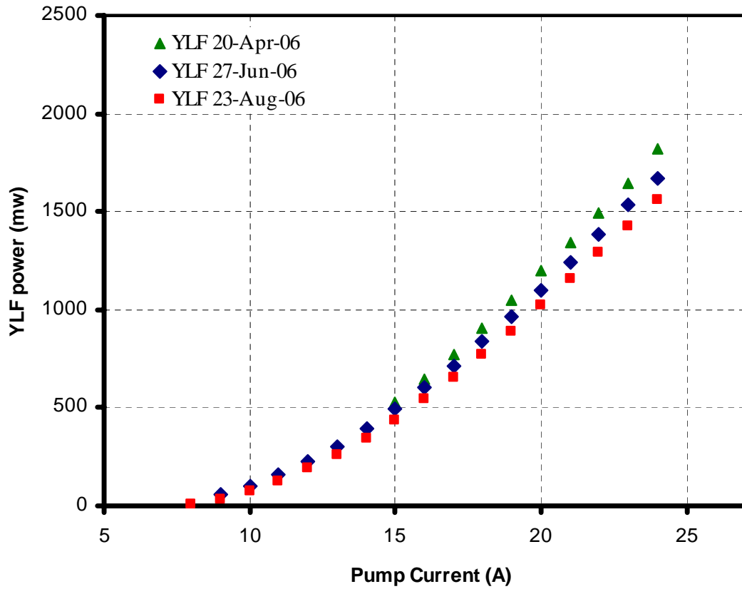
Nd:YLF LASER PUMPED TI:S LASERS 2
